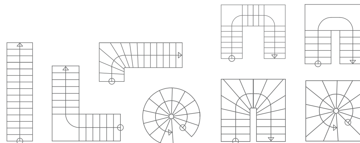
Grundrissvarianten
